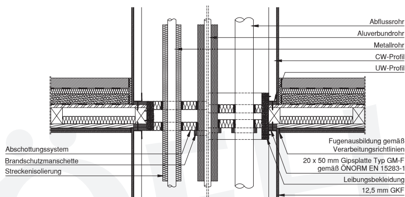
Bild 11: Ausbildung einer horizontalen Abschottung im Bereich einer Holzrahmendecke (Schachttyp B)
