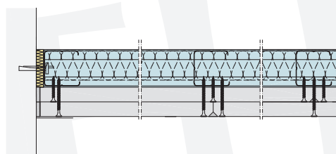
Bild 14: Wandanschluss an Massivwand
