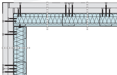
Bild 16: Eckausbildung Schachtwand
