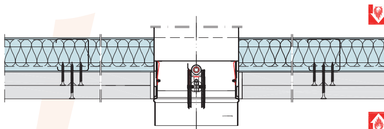
Bild 6: Feuerschutzabschluss FLI-VE
