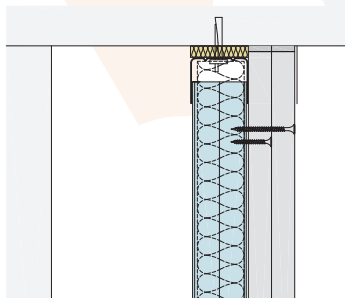
Bild 15: Deckenanschluss an Massivdecke
