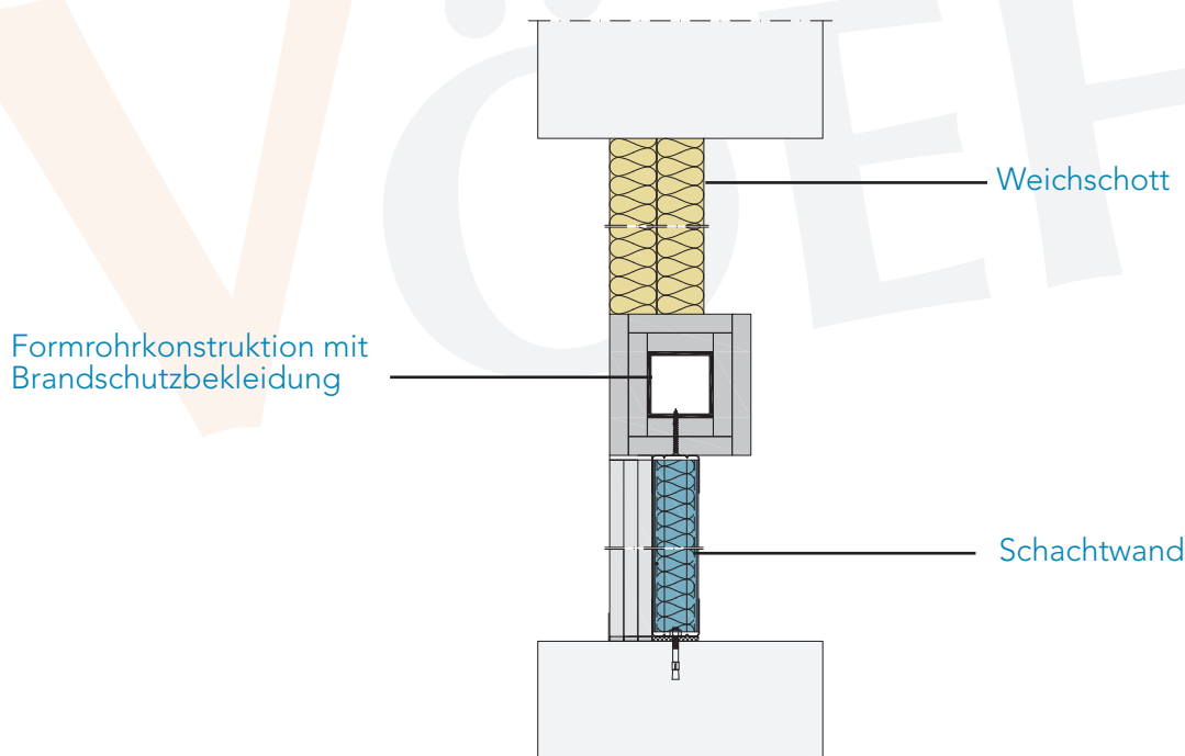
Bild 7: Schachtwand mit Weichschott gemäß ÖNORM H 6031
